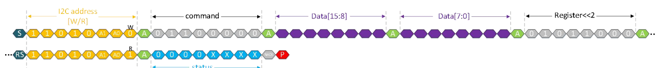
图 15-7. 写寄存器 I2C 时序图
