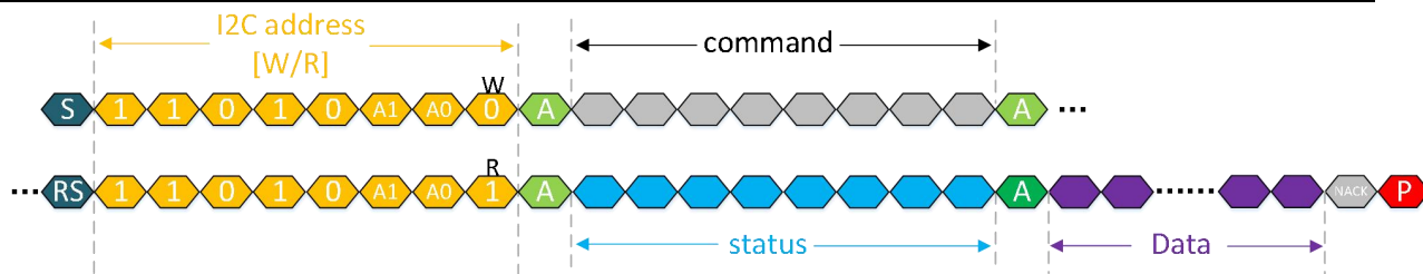
图 11-2. 测量数据回读帧 I2C 通信示意图
