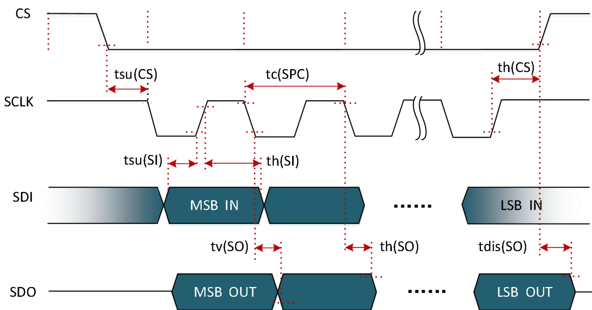
图 12-1 SPI 时序图
