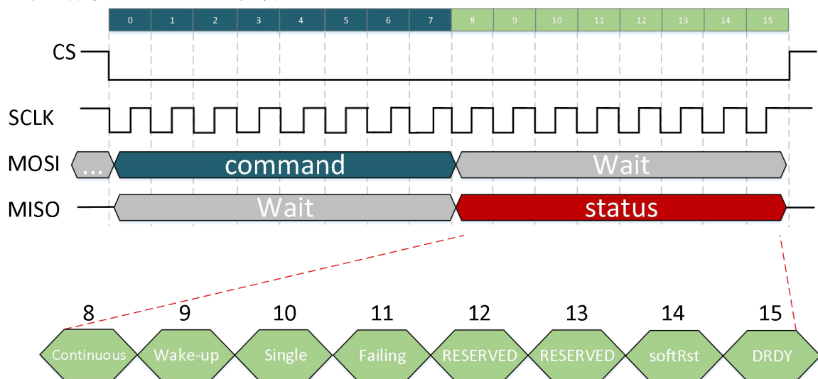
图 10-1. 芯片运行状态 SPI 说明
