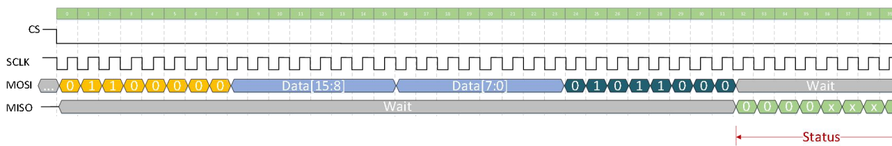
图 15-4. 写寄存器 0x16 SPI 时序图
