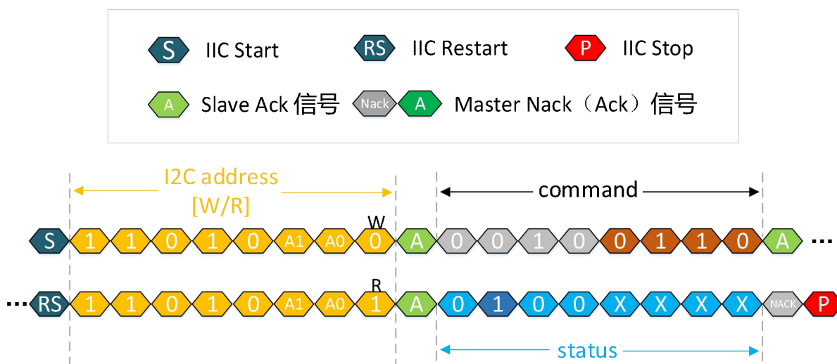
图 8-4. 唤醒睡眠模式 I2C 通信图
