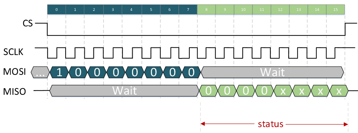
图 8-7. 空闲模式 SPI 通信图
