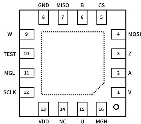
图 3: QFN-16L 3mmx3mm
