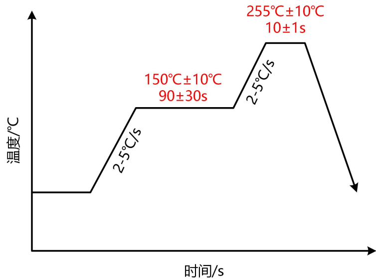
图 22: 焊接温度曲线
