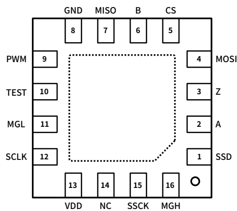
图 3: QFN-16L 3mmx3mm
