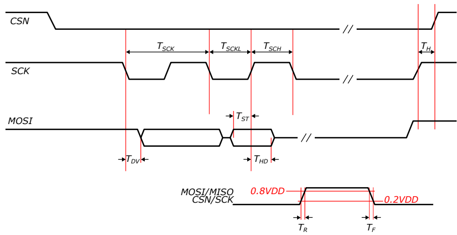
图 8: SPI 时序图
