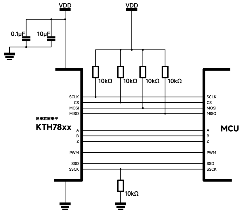
图 2: 应用电路
