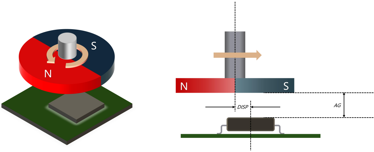
图 5: 在轴磁铁芯片摆放位置
